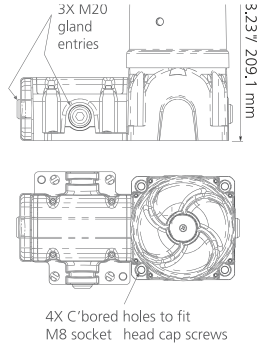
Montage en saillie Ex de représenté
