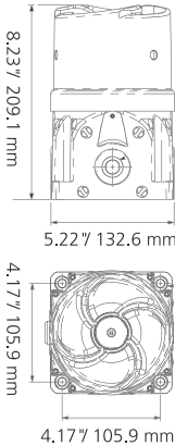
Montage en saillie Ex d représenté
